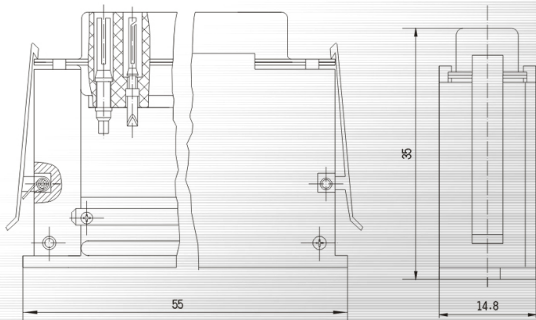
带护线壳的自动锁紧型高低频混装连接器 DB17S2GS1T 型
