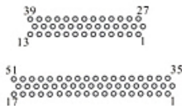
J40系列插针连接器孔位排列图
