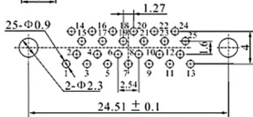
印制板开孔尺寸
