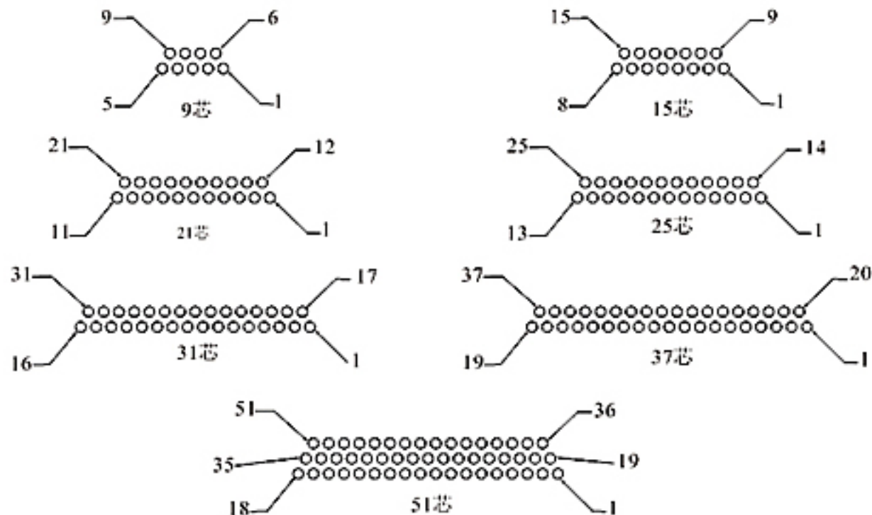
12.CDbA系列插头连接器孔位排列图（从对插面看）
