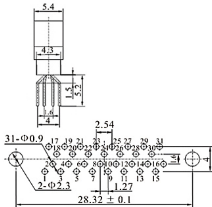
印制板开孔尺寸
