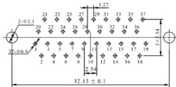
印制板开孔尺寸
