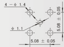
安装开孔尺寸 Mounting hole
