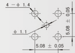
安装开孔尺寸 Mounting hole
