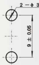
安装开孔尺寸 Mounting hole
