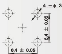
安装开孔尺寸 Mounting hole
