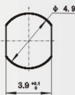
安装开孔尺寸 Mounting hole
