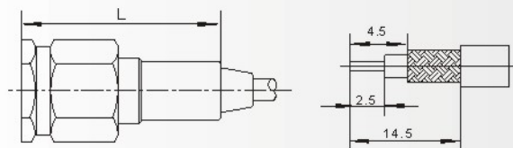
电缆剥线尺寸 Cable stripping dimensions
