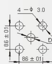
安装开孔尺寸 Mounting hole
