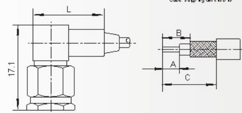
电缆剥线尺寸 Cable stripping dimensions
