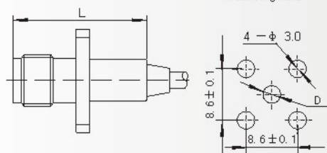
安装开孔尺寸 Mounting hole
