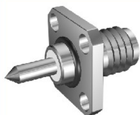
SMA-KFD183
