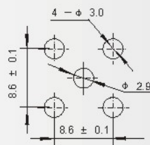
安装开孔尺寸 Mounting hole
