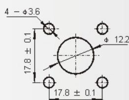
安装开孔尺寸 Mounting hole
