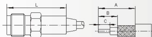
电缆剥线尺寸 Cable stripping dimensions
