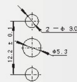
安装开孔尺寸 Mounting hole
