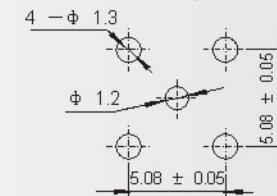
安装开孔尺寸 Mounting hole
