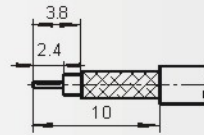
电缆剥线尺寸 Cable stripping dimensions
