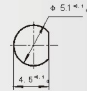
安装开孔尺寸 Mounting hole
