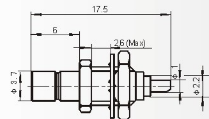
安装开孔尺寸 Mounting hole
