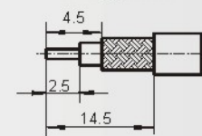
电缆剥线尺寸 Cable stripping dimension
