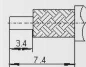
电缆剥线尺寸 Cable stripping dimensions
