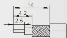
电缆剥线尺寸 Cable stripping dimensions
