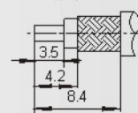
电缆剥线尺寸 Cable stripping dimensions
