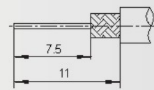
电缆剥线尺寸 Cable stripping dimensions
