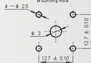
安装开孔尺寸 Mounting hole
