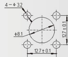
安装开孔尺寸 Mounting hole
